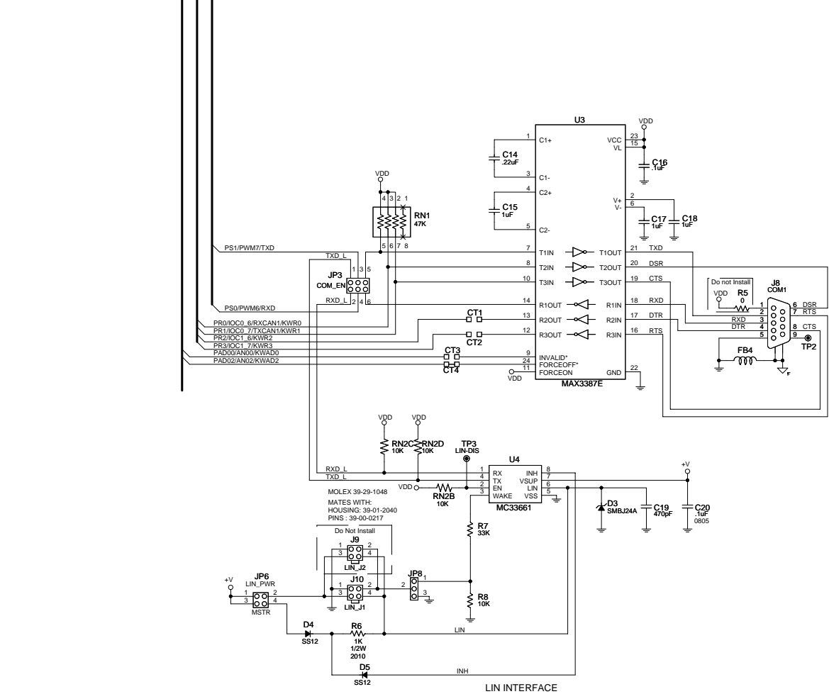
LIN INTERFACE
